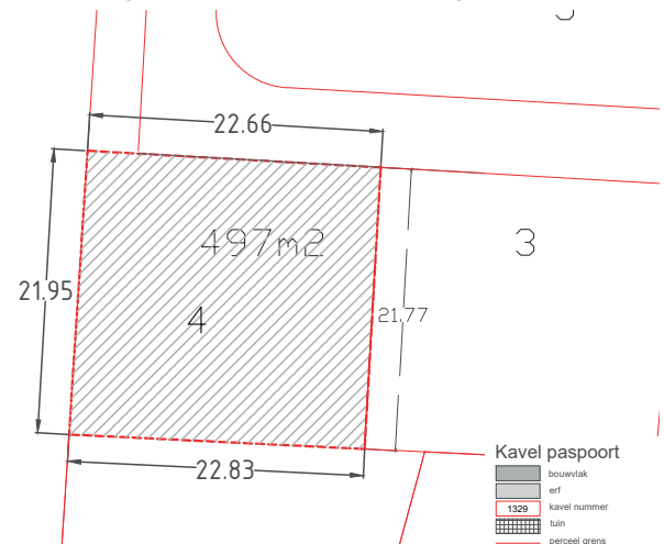
afb. 3 | Bestemmingsplanfunctie en maatvoering
